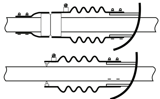
joint d'arbre étanche
