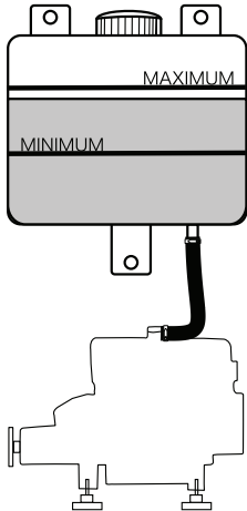
bouteille de trop-plein
