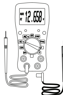
multimètre
